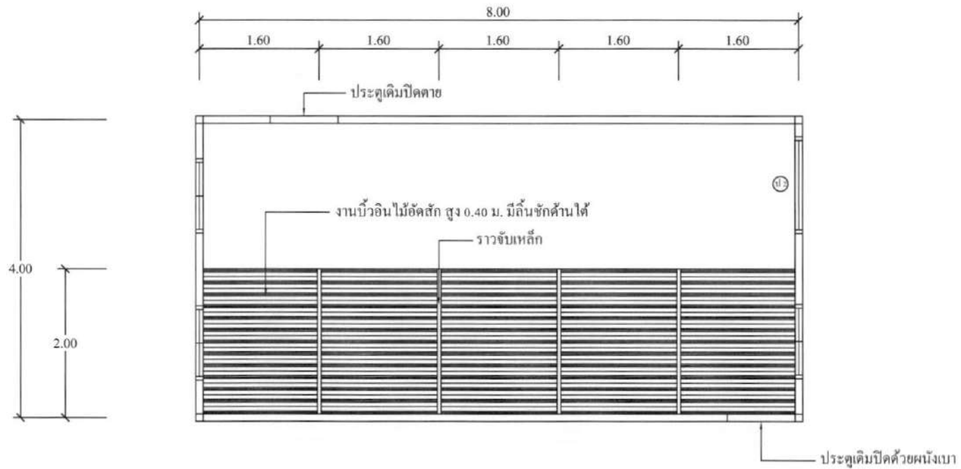
แบบขยายห้องนวดแผนไทย มาตราส่วน 1 : 100
