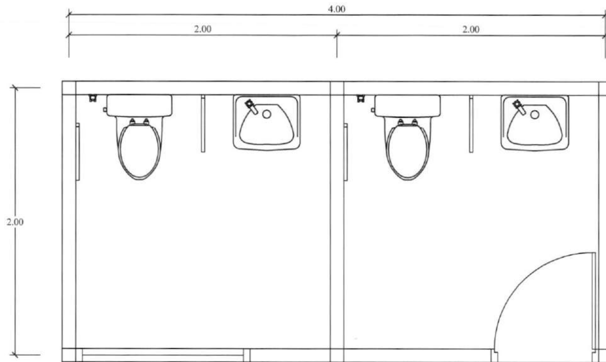
แบบขยายห้องน้ำ มาตราส่วน 1 : 20
